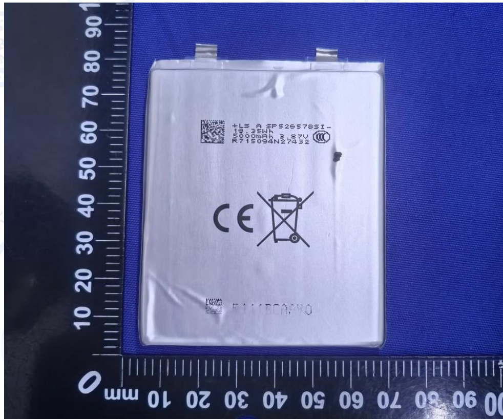
Photo 3 内部电芯 Internal Cell
