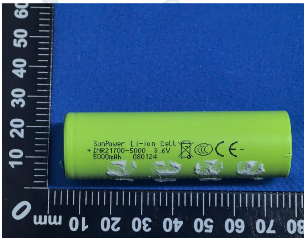
Photo 4 Internal Cell 内部电芯
