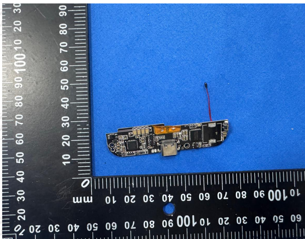
Picture 8. Back view of protection board 图片 8. 保护板后视图
