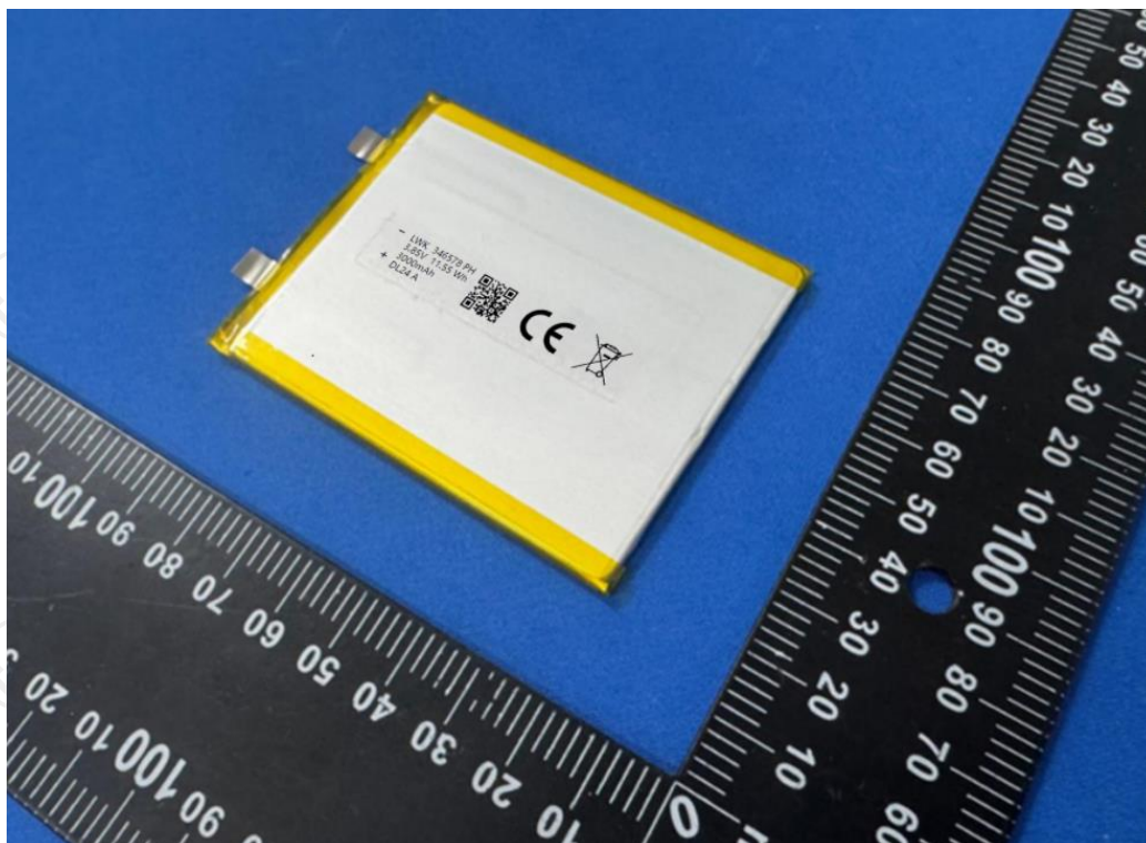
Picture 5. Front view of cell 图片 5. 电芯前视图
